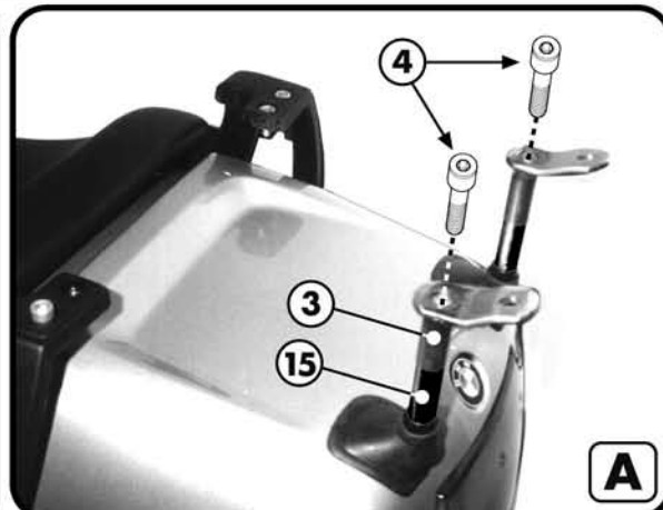
VITE TCEI M6x20mm SCREW M6x20mm VIS M6x20mm SCHRAUBE M6x20mm TORNILLO M6x20mm
